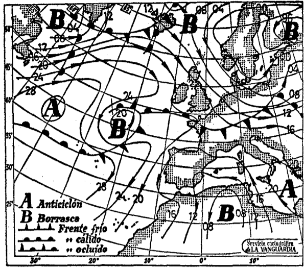
La borrasca de Argelia seguirá determinando alguna inestabilidad atmosférica en la región catalana.
