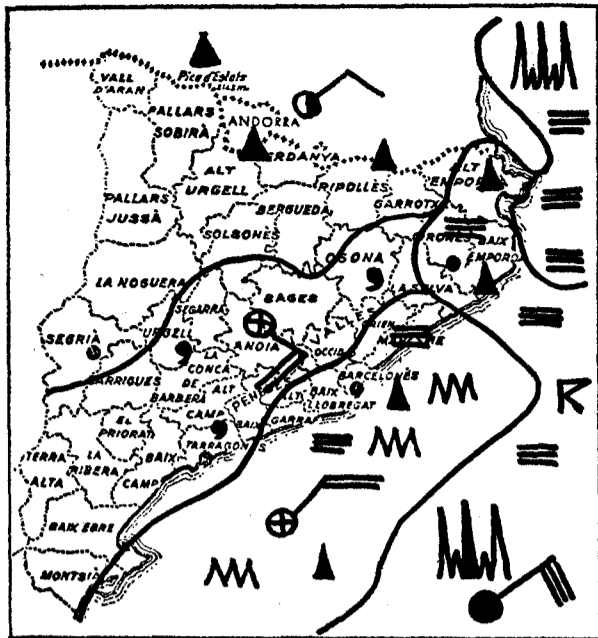
La borrasca de Argelia seguirá determinando alguna inestabilidad atmosférica en la región catalana.
